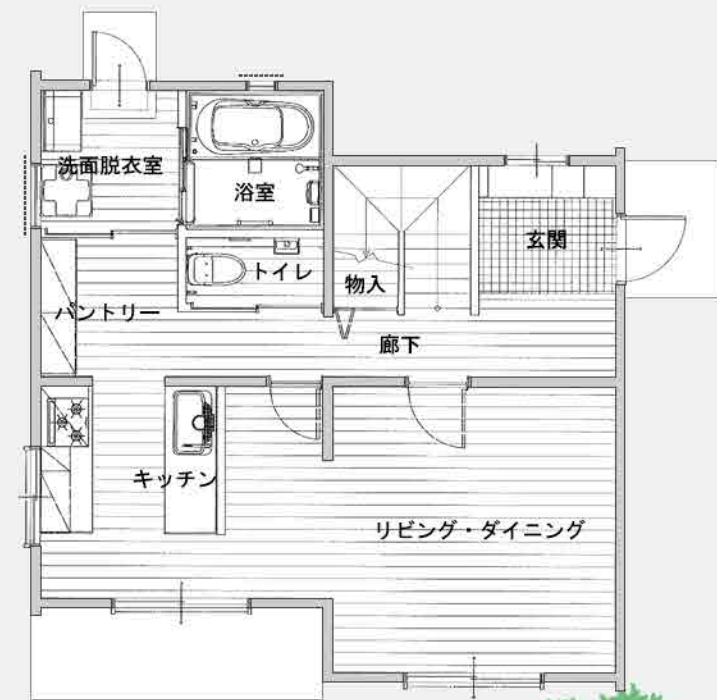
施工後：1階平面図
