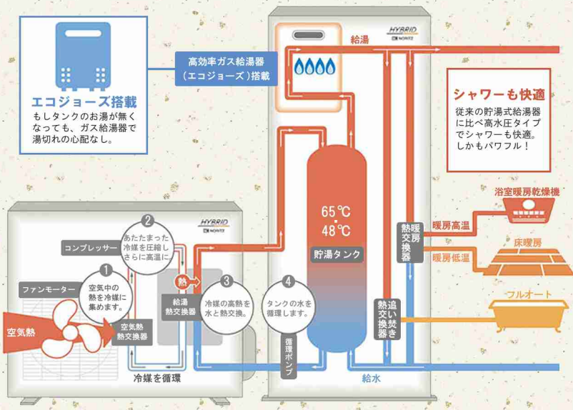
ヒートポンプユニット内部
